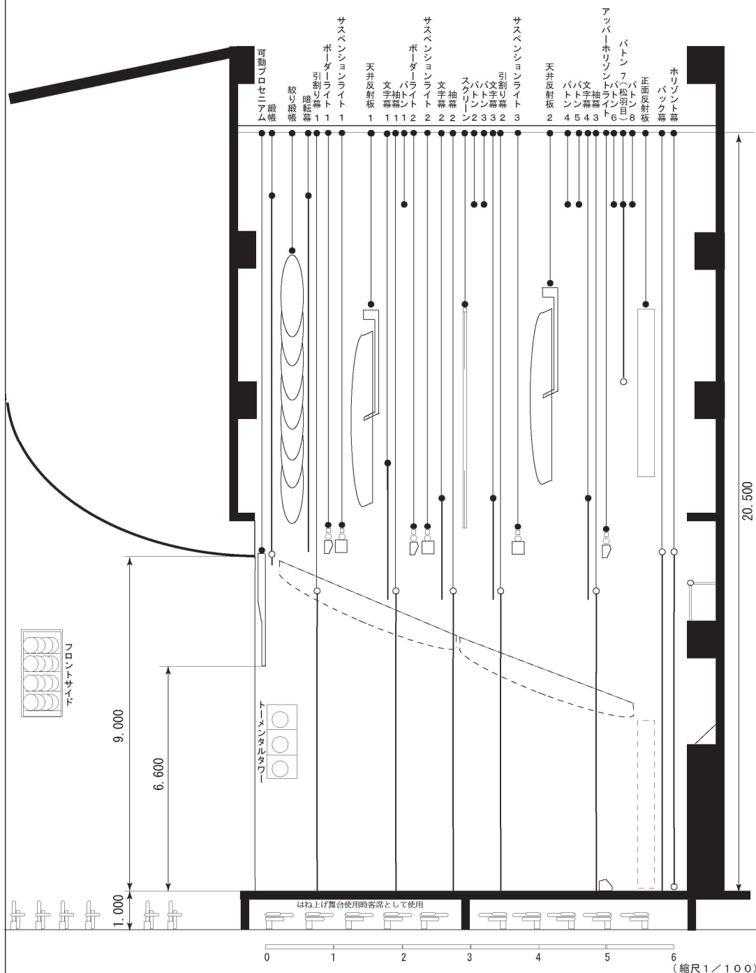
広島県民文化センターふくやま 舞台断面図
